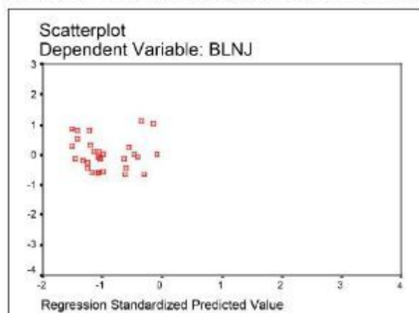
Grafik 1 Scatterplot
